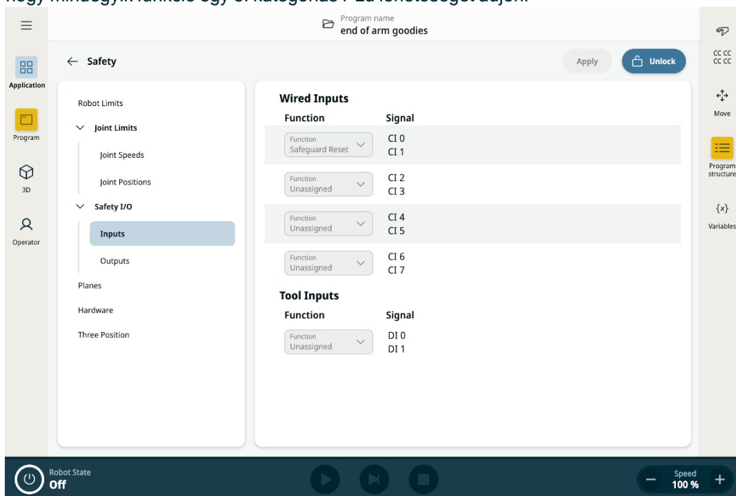
Ábra 1.4 : A PolyScope X képernyője a megjelenített bemeneti jelekkel.
